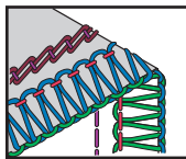
Zajišťovací steh s 5 nitěmi 12 mm nebo 16 mm na sešívání a začísťování pevných materiálů.
