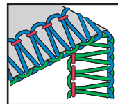
Overlockový steh se 3 nitěmi široký nebo úzký , tento začísťovací steh je vhodný na veškeré materiály.
